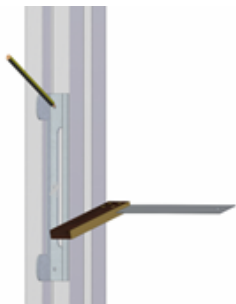
Schließblech bündig an Vorderkante anlegen ...
