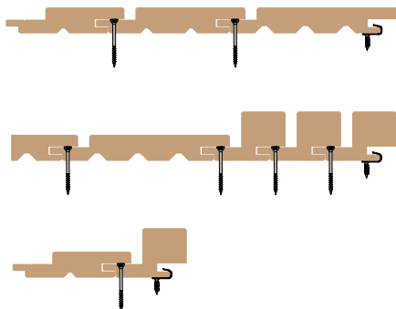
Fassadenprofil Verto
